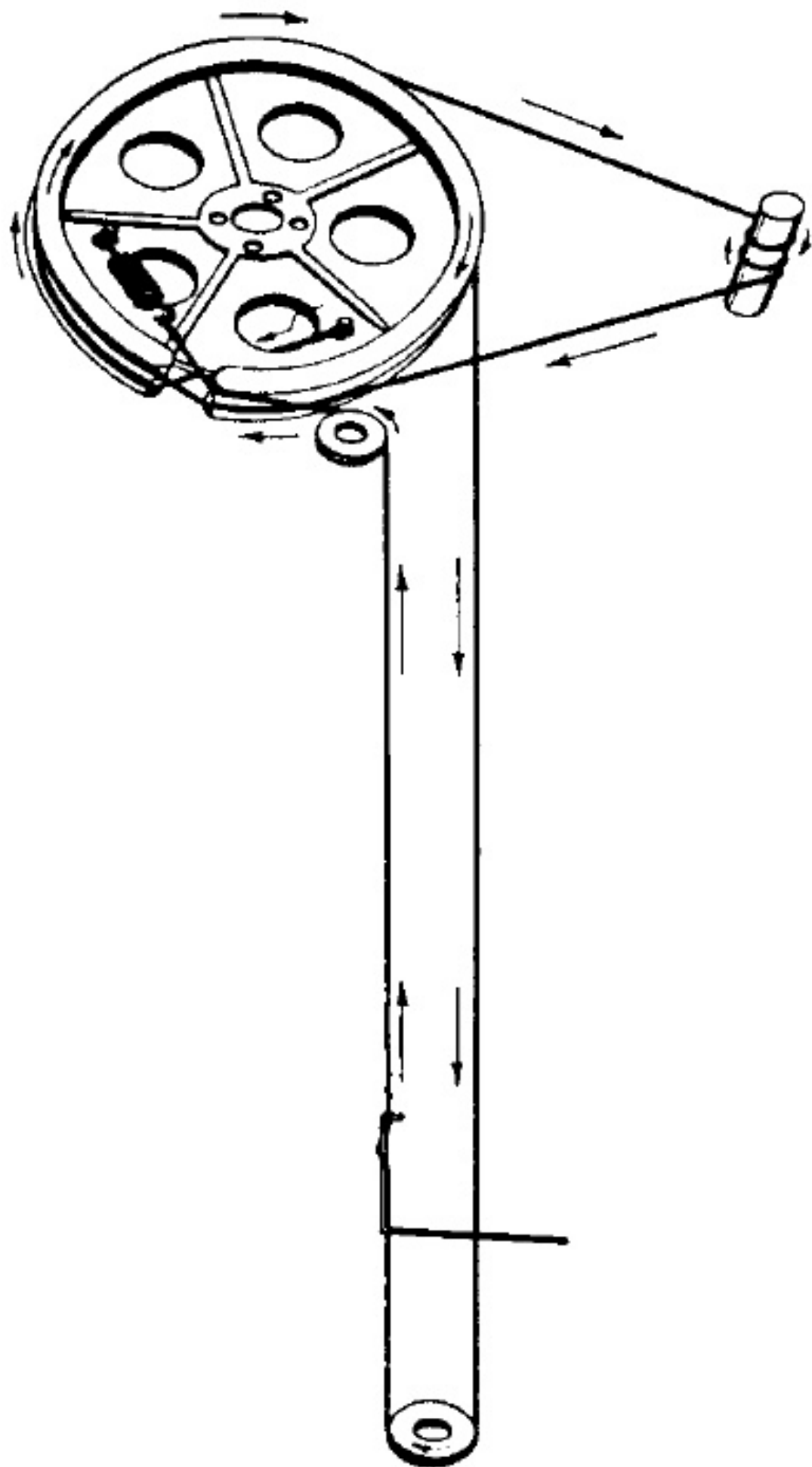
SCHEMA PER IL MONTAGGIO DELLA FUNICELLA
